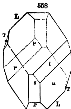
Dauphiny.
